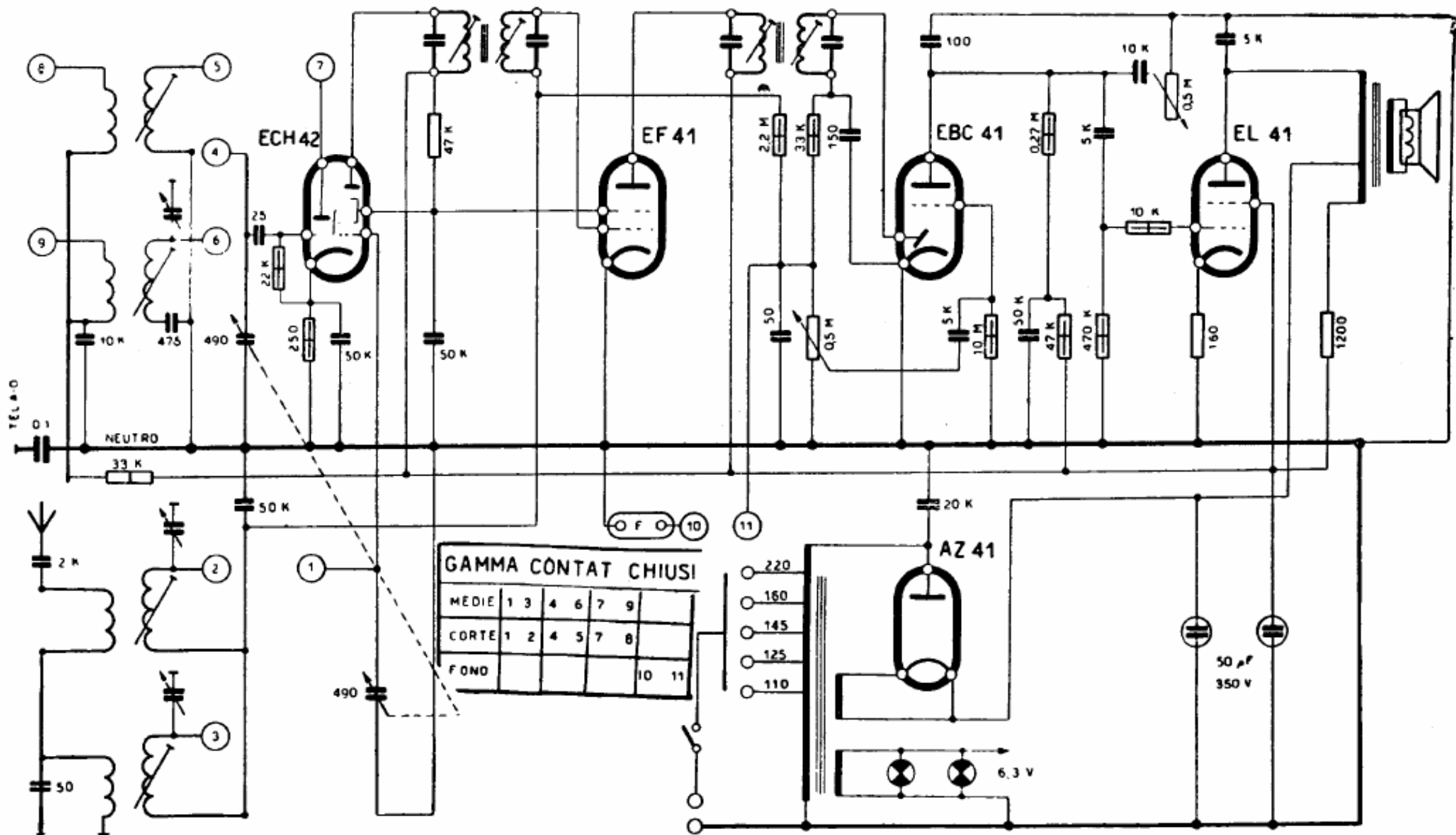
VEGA - Mod. 622. Onde medie da 520 a 1620 kc/s. Punti di taratura 580-1500 kc/s. Onde corte da 5,6 a 18 Mc/s. Media frequenza 470 kc/s. Potenza indistorta di uscita 2,5 watt. Consumo 42 watt.
